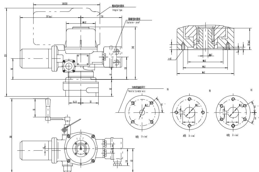
QB2, QB2Ex 法兰连接型式尺寸
