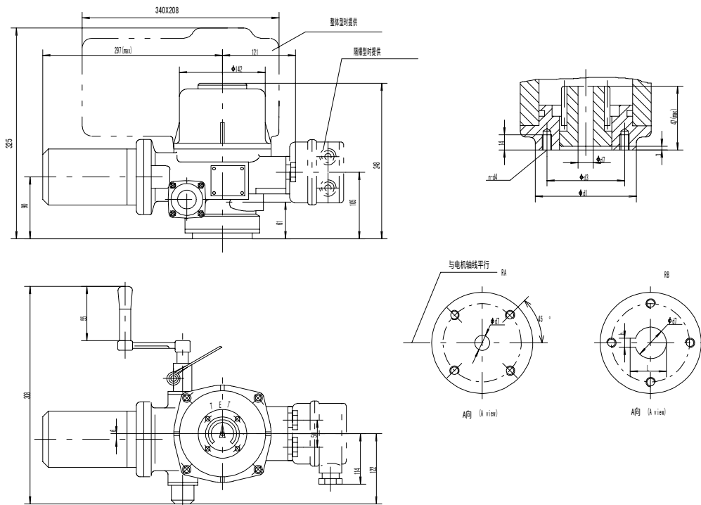
QB1, QB1Ex 法兰连接型式尺寸
