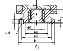
QBR3法兰结构、型式及尺寸表
