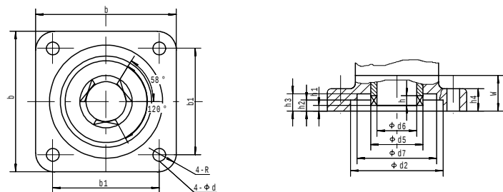
方形法兰连接尺寸
