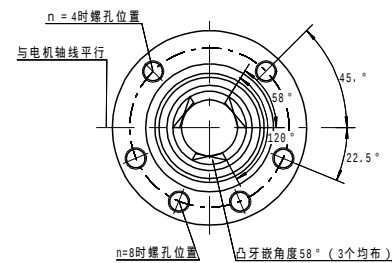
ISO标准法兰连接尺寸
