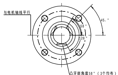
JB2920-81法兰连接尺寸
