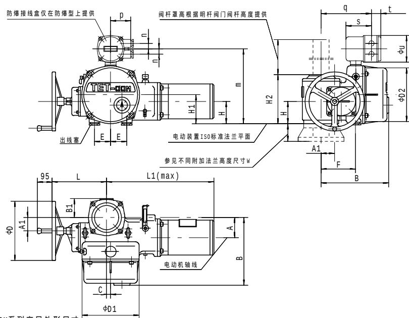
00M系列产品外形尺寸
